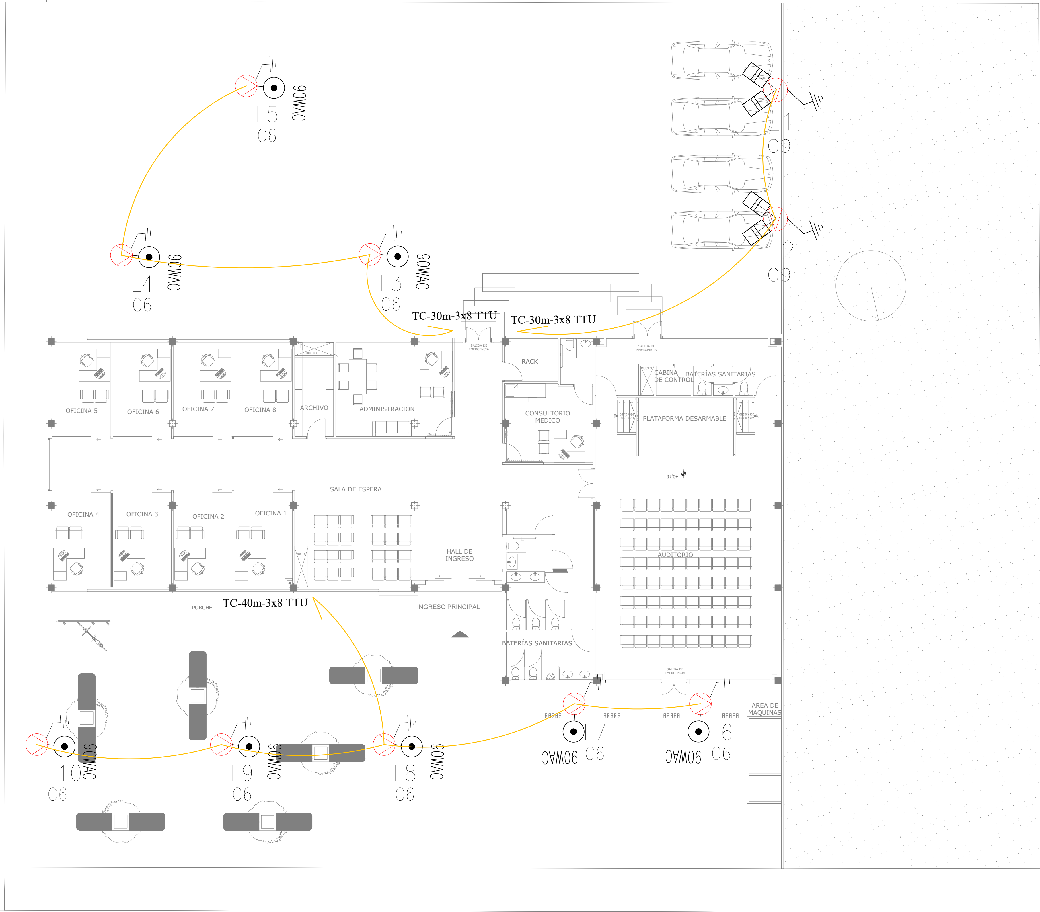
CALLE EUGENIO NICOLAS PALMA MOREIRA CIRCUITO ILUMINACION EXTERIOR ESCALA 1:100
